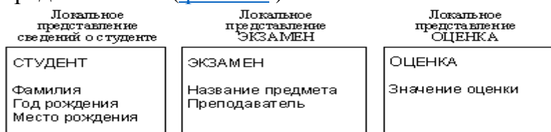
Рис. 5.5. Локальные представления
